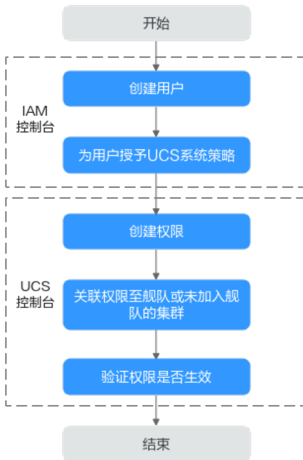
图 5-5 给用户授予 Kubernetes 资源权限流程
