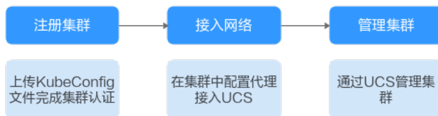
图 1-14 附着集群管理流程
