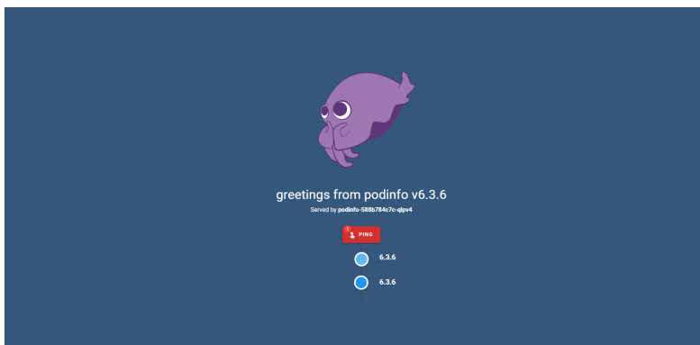
图 7-2 Podinfo 界面
