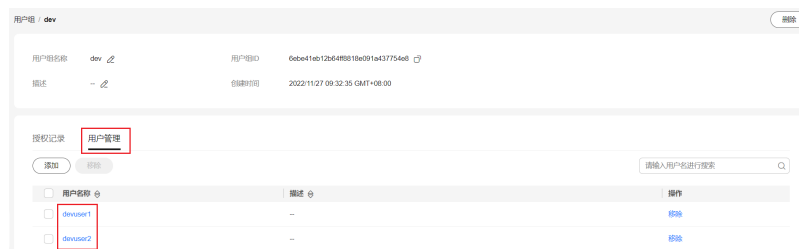
图 5-13 用户管理
