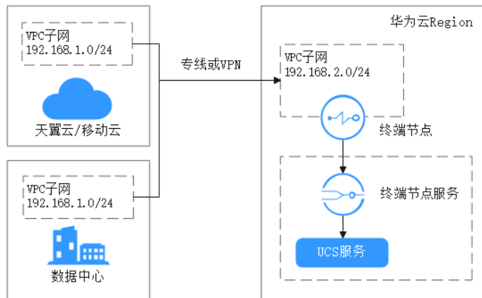
图 9-8 私网接入原理
