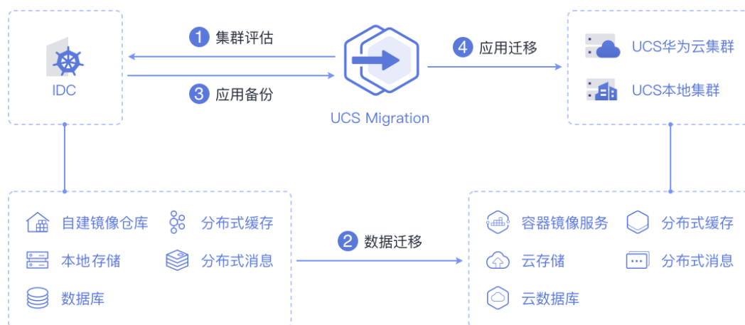
图 10-1 迁移流程
