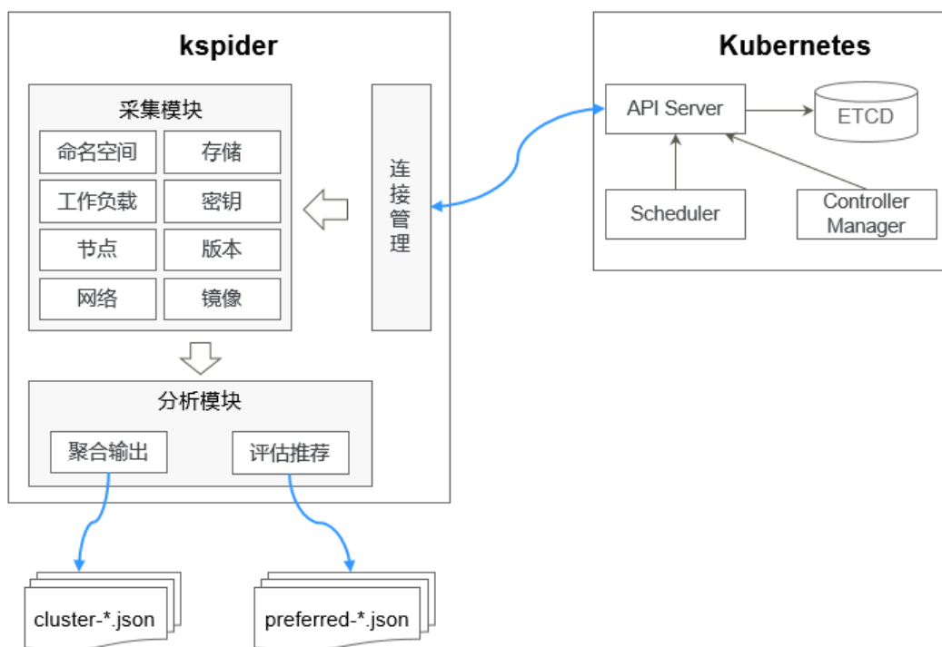
图 10-12 kspider 架构
